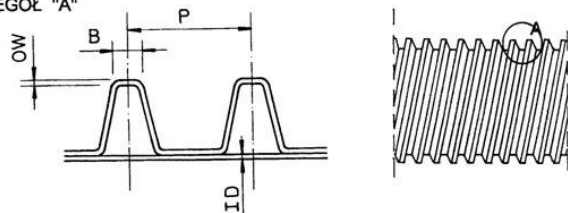
Rys. 1. Karby na rurze polietylenowej
