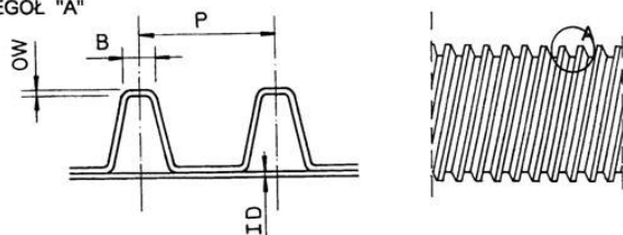
Rys. 1. Karby na rurze polietylenowej
