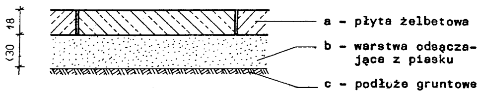
Rys. 2. Przykładowy przekrój poprzeczny nawierzchni z płyt
